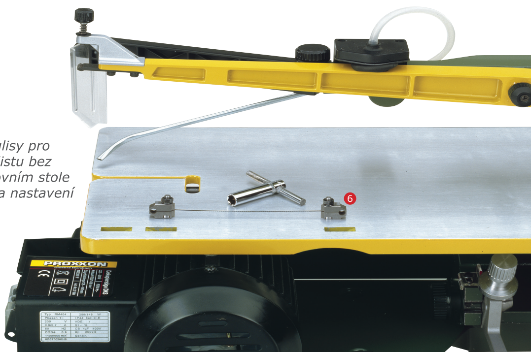
6 Upínací kulisy.
