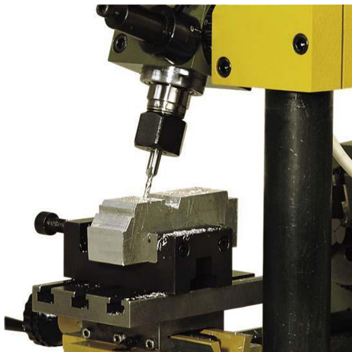
Svěrák PM 60 na křížovém stole s T-drážky.
